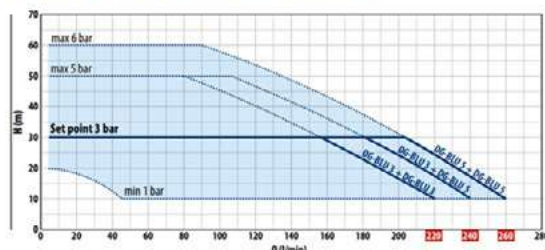
CURVAS DE PRESTACIONES DE UN GRUPO DE DOS UNIDADES DG-BLU
