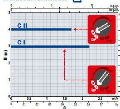
CURVAS DE PRESTACIONES ΔC
